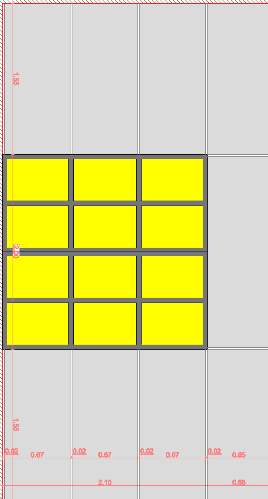
Σχέδιο 1 : Όψη Διαχωριστικού Τοίχου
